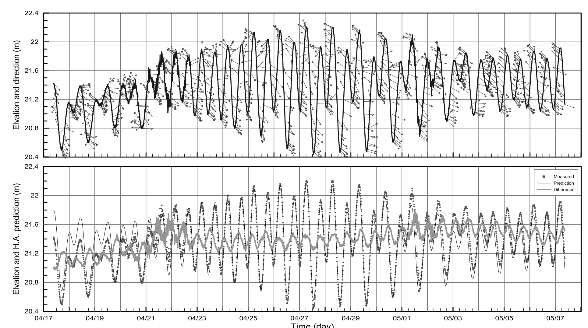
潮位實測紀錄 (套繪流向)
