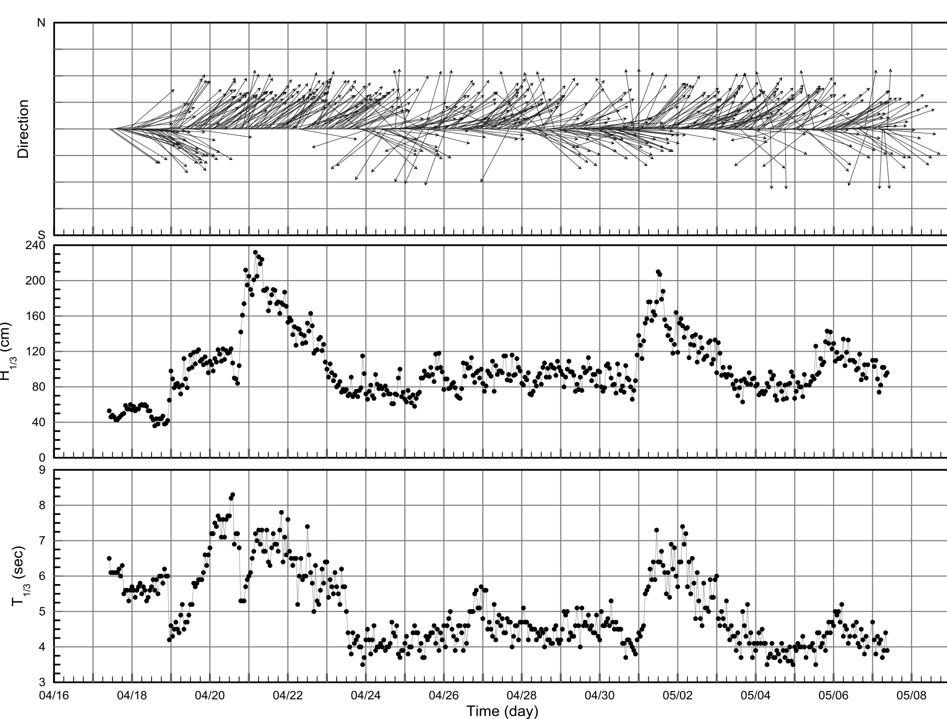
波浪實測紀錄
