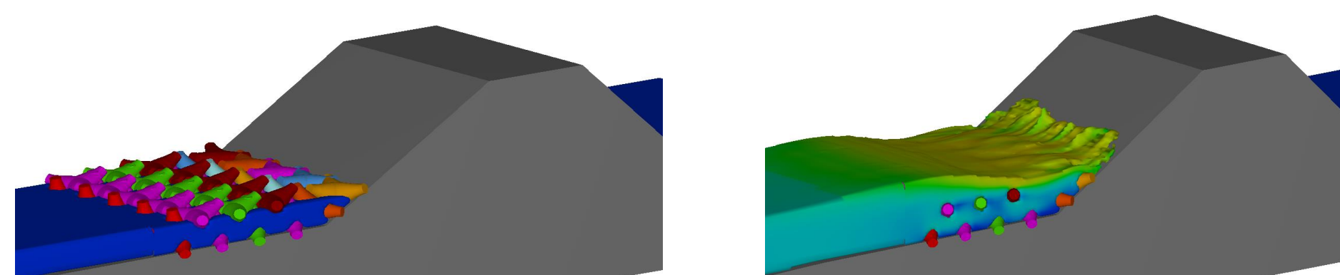
波浪溯升與堤頭流沉 (Flow-3D)
