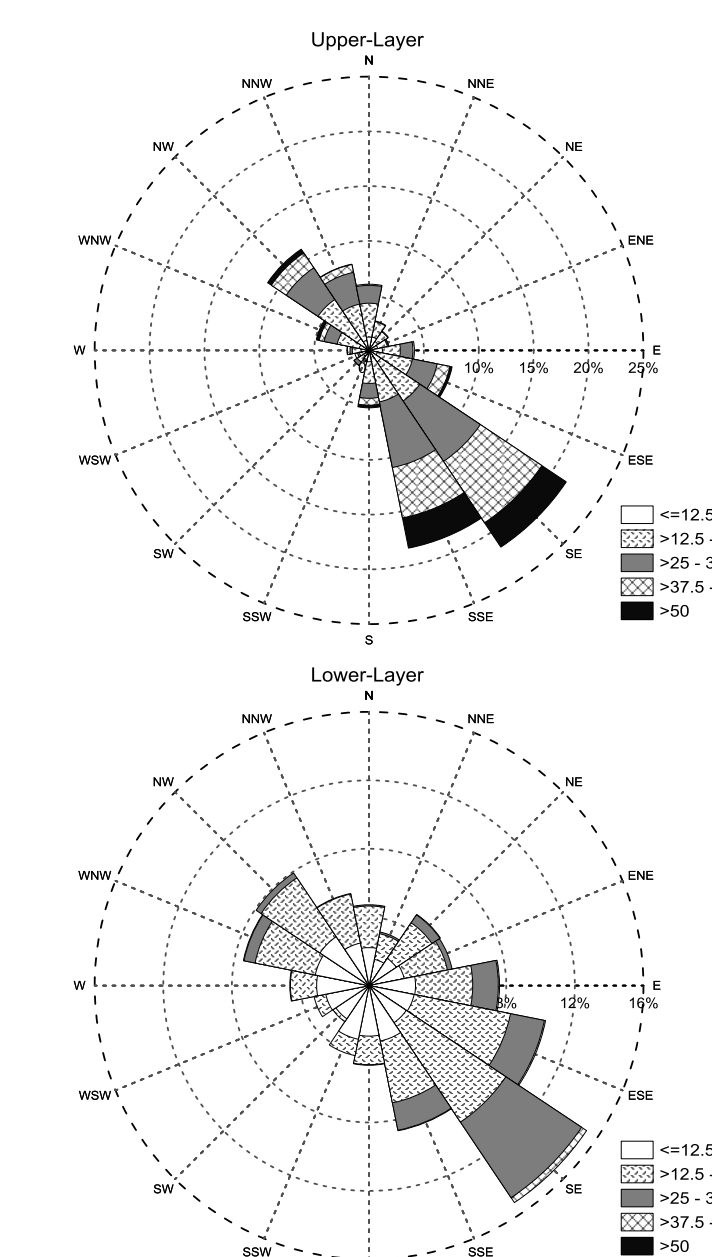
流速流向玫瑰圖
