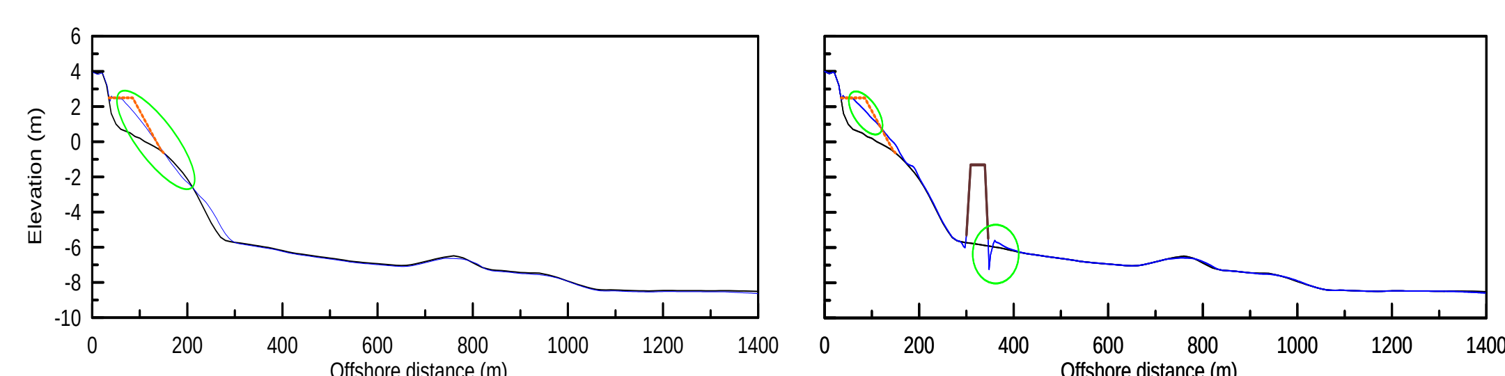
海灘斷面侵蝕 (SBEACH)
