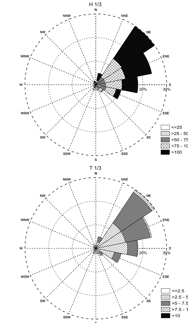
波高波向玫瑰圖
