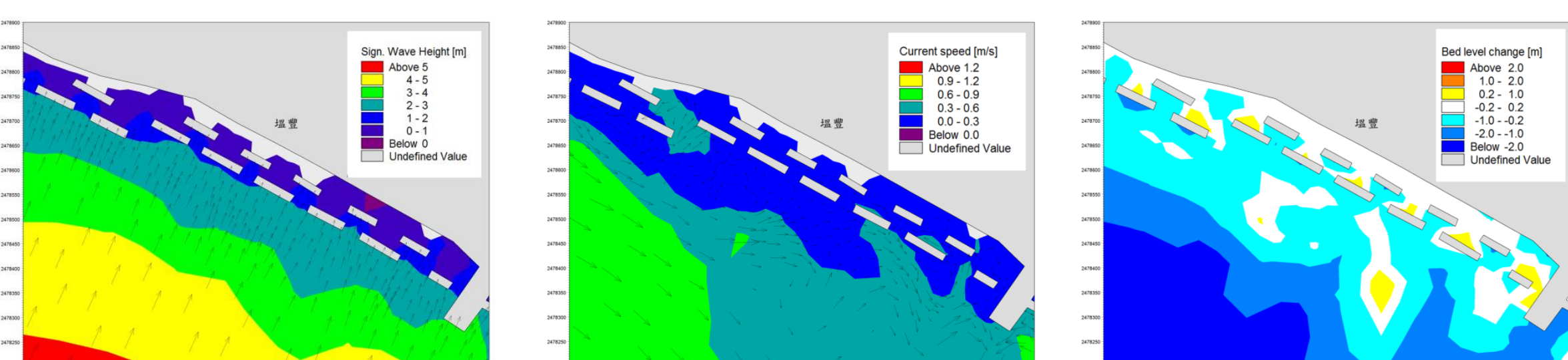
波流地形變化 (MIKE21)
