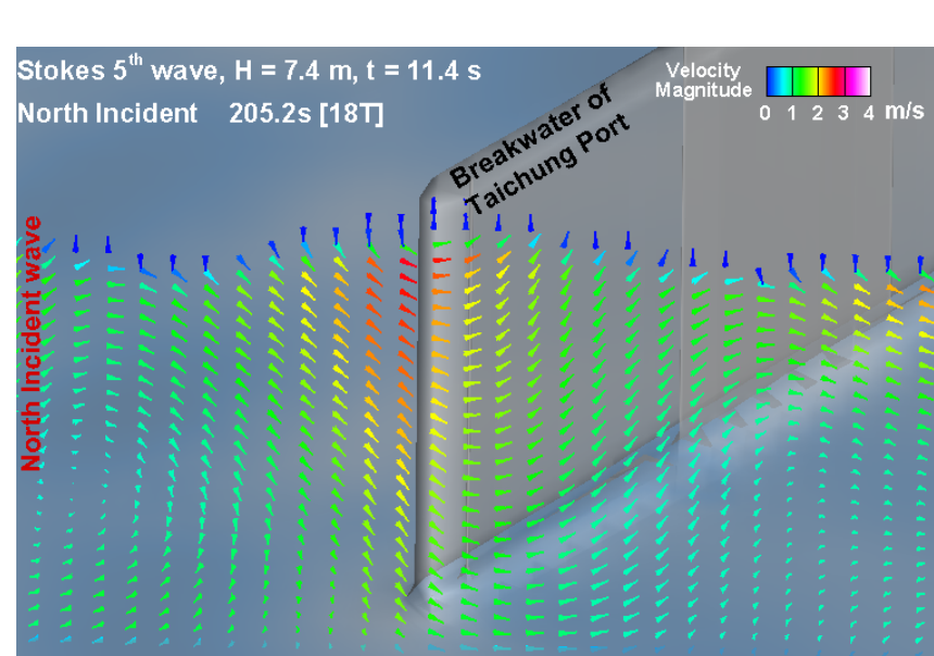
波浪溯升與堤頭流沉 (Flow-3D)
